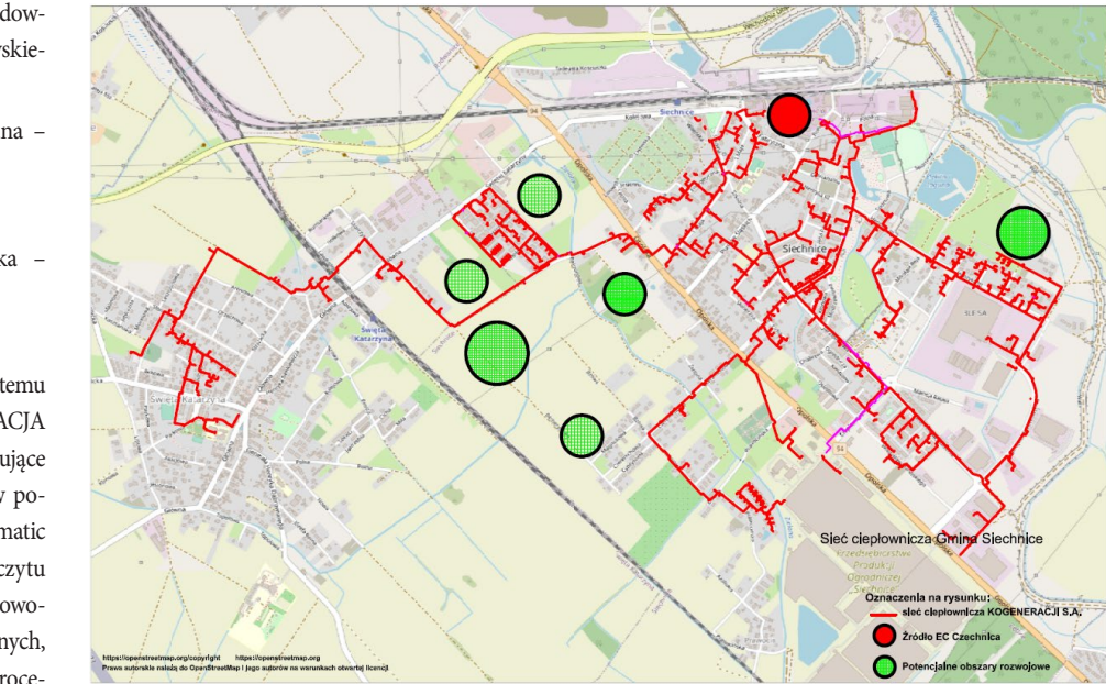
Mapka z aktualnym stanem sieci ciepłowniczej w Gminie Siechnice oraz potencjalnymi obszarami rozwojowymi.
